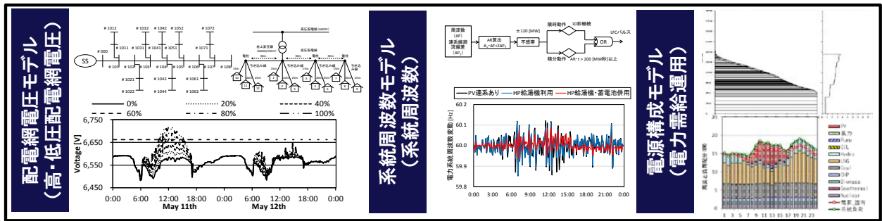
図1 エネルギーマネジメントシステム性能評価モデルの全体像
