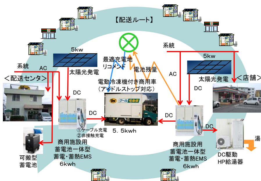
図-1: 蓄電池付き商用施設向け蓄電・蓄熱EMSと冷凍機付き商用車(アイドルリングストップ対応)との連携システム全体像
